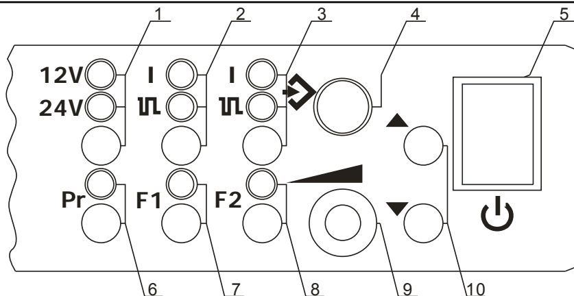
Рисунок 6. Панель управления устройством
