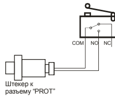
Рисунок 11. Схема подключения защитных концевиков
