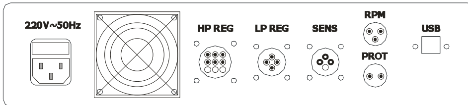
Рисунок 4. Задняя панель
